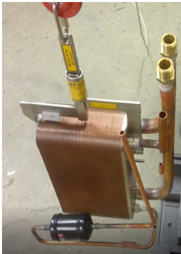
Ett litet mekaniskt klämverktyg för hantering av värmeväxlare
